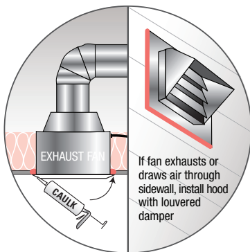
17 Exhaust Fan
